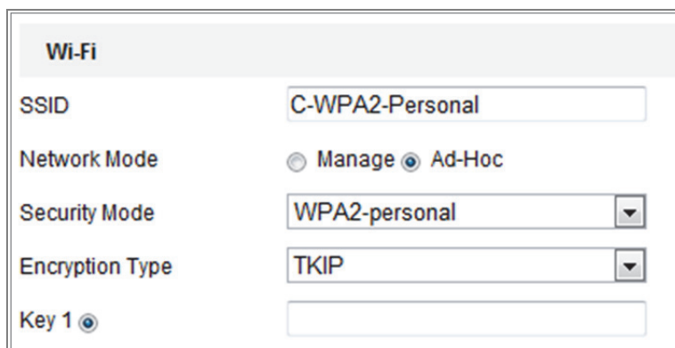
Obrázek 4-3 Nastavení sítě Wi-Fi - režim ad hoc
